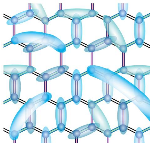
図 2: ランダムシングレットの概念図。Zn(hfac) 2 (A x B 1-x ) 結晶中の乱れを持つハニカム格子上で、青丸のスピスがランダムなパターンでペアを組み、非磁性の量子状態を形成している。
