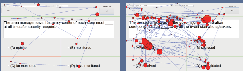
図2・3：視線を用いた確信度推定
